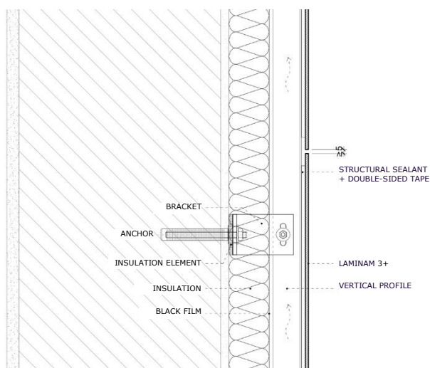
Вертикальный разрез
